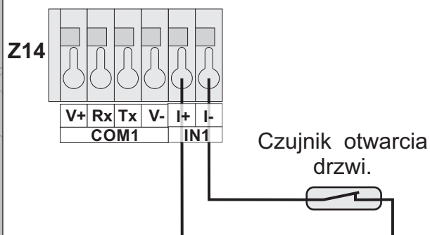
Schemat podłączenia czujnika otwarcia drzwi.
