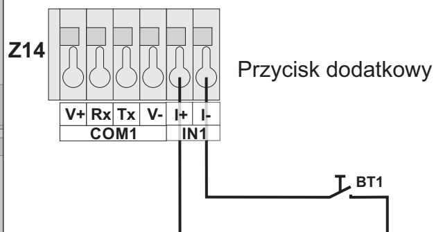
Schemat podłączenia wejścia DIN
